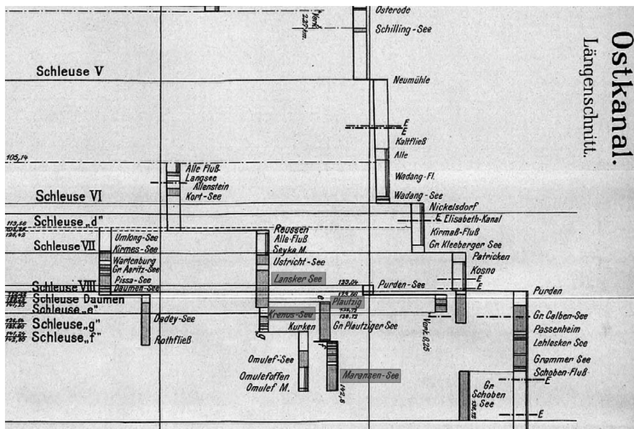
Rozmieszczenie śluz pomiędzy jeziorami Łańsk, Pluszne, Kiernoż, Maróz
